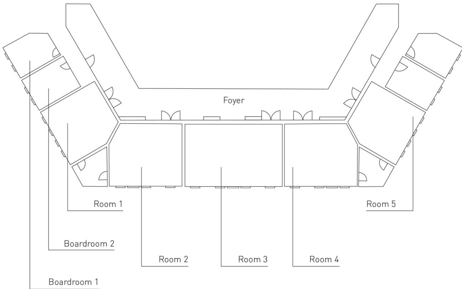
Grundriss Tagungsräume
